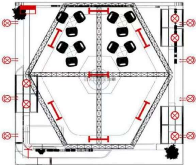
电气平面图 Electrical Plan
